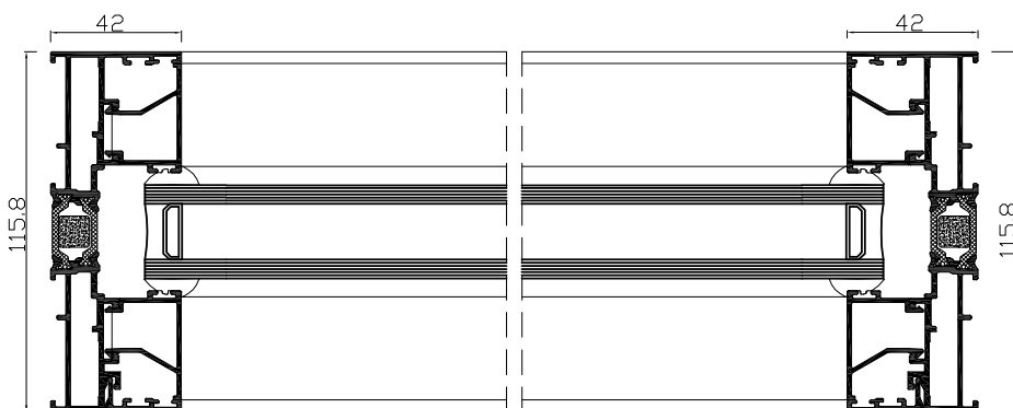
PRZEKRÓJ A-A
