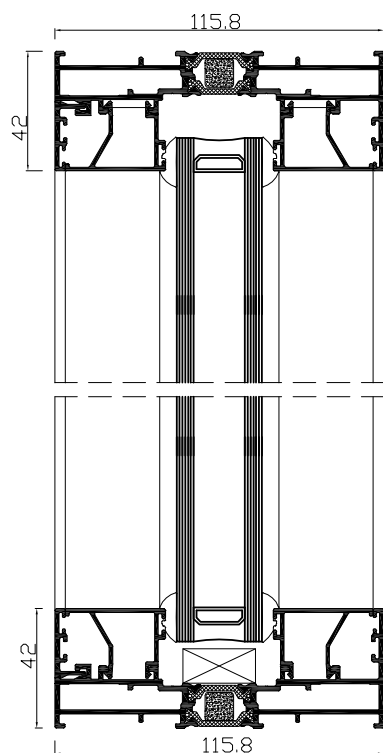
PRZEKRÓJ B-B
