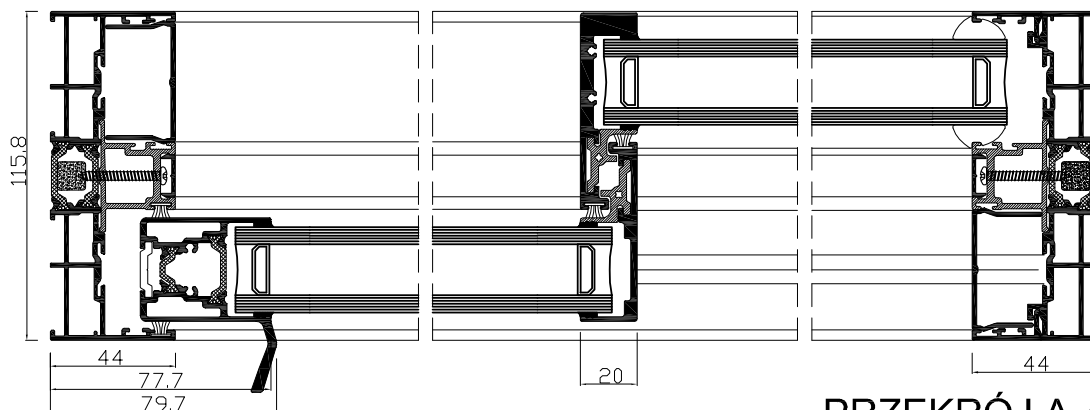
PRZEKRÓJ A-A
