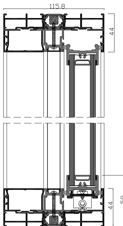
PRZEKRÓJ C-C
