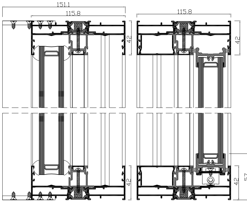
PRZEKRÓJ C-C
