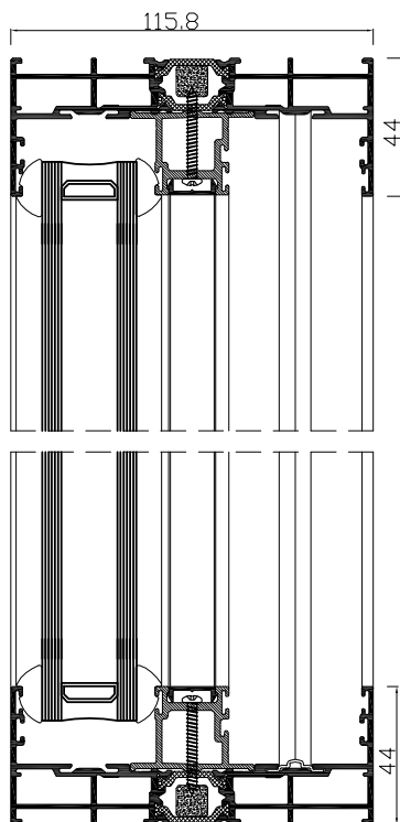
PRZEKRÓJ B-B
