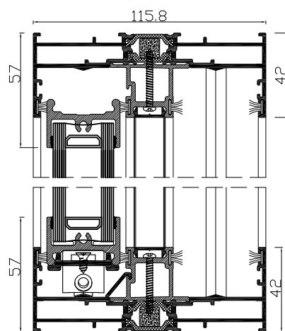
PRZEKRÓJ B-B
