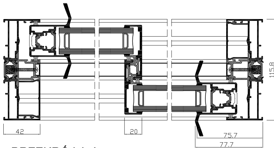
PRZEKRÓJ A-A
