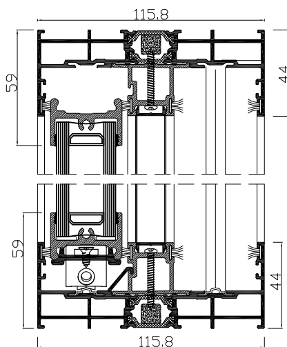
PRZEKRÓJ B-B
