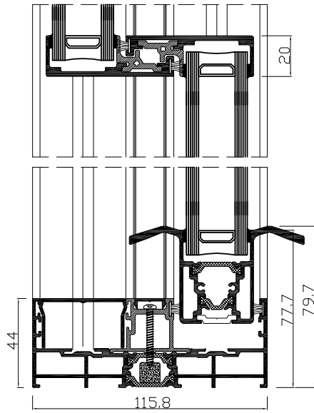
PRZEKRÓJ A-A
