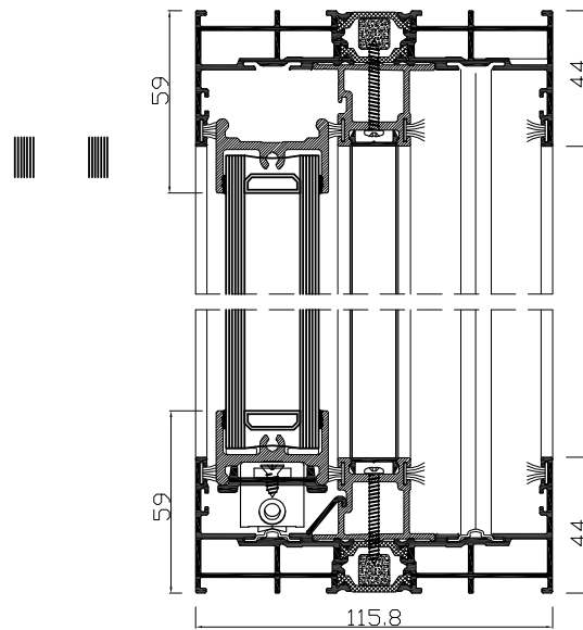
PRZEKRÓJ B-B
