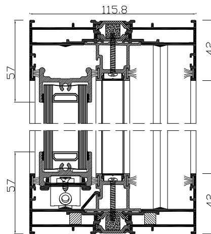
PRZEKRÓJ B-B
