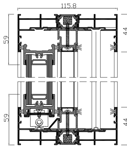
PRZEKRÓJ B-B
